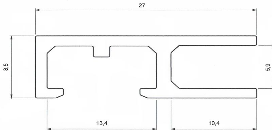
Rückrahmen Profil 9
