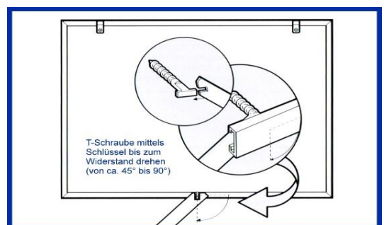
Sicherung mit T-Schrauben
